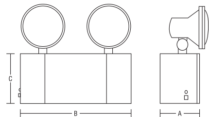
Dimensions (in,mm.)
